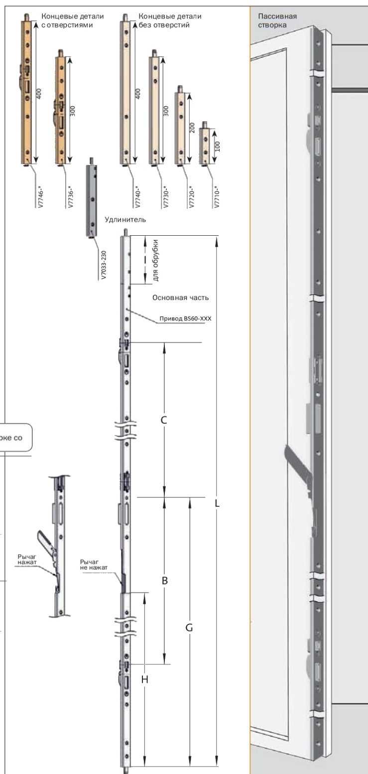
Схема монтажа для серии BS60-733-2
