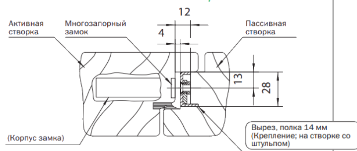
Схема монтажа для серии BS60-280
